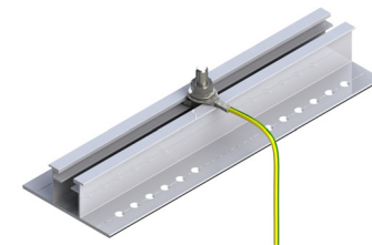
Befestigung des Erdungdrahts mittels Hammerkopfschraube
